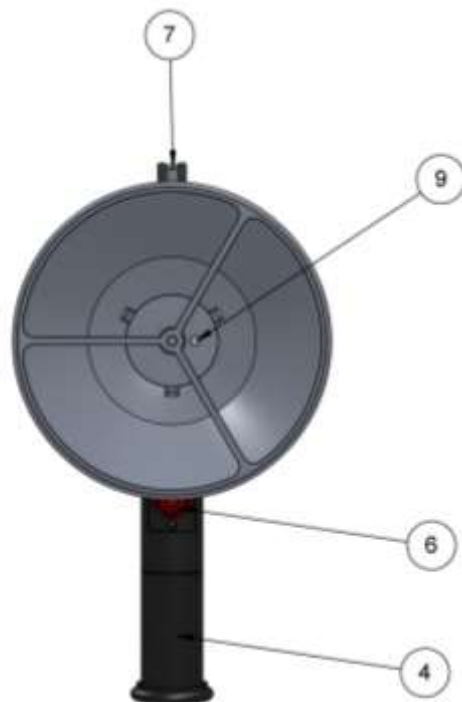
Рис. 3. Имитатор пламени (вид спереди)
